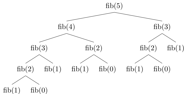
Abbildung 4.3: Die Anzahl Funktionsaufrufe für F(5) ist 15.
