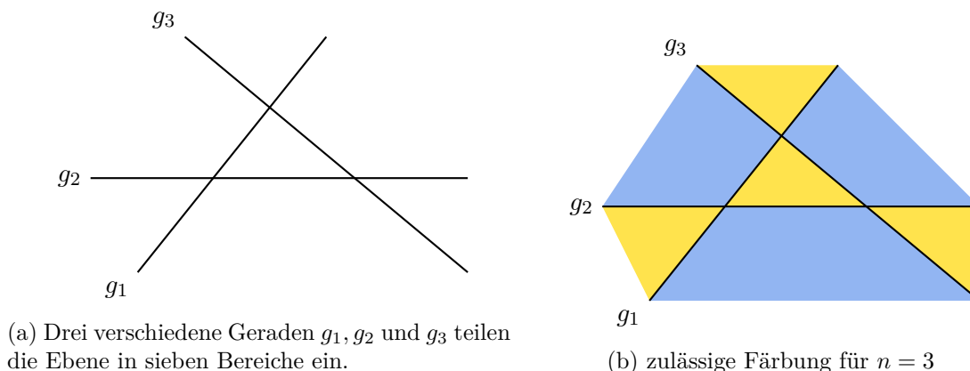
Abbildung 3.4: zulässige Färbung für drei Geraden
