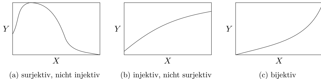
Abbildung 1.1: schematische Darstellung der Eigenschaften in Definition 1.3
