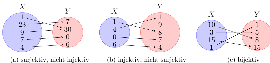
Abbildung 1.2: Diagramm-Darstellung der Eigenschaften in Definition 1.3
