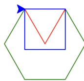
Programm 4.3: farb_vieleck.py
