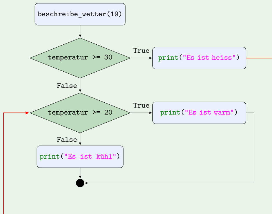
Abbildung 5.2: Flussdiagramm für den Code aus Aufgabe 5.7
