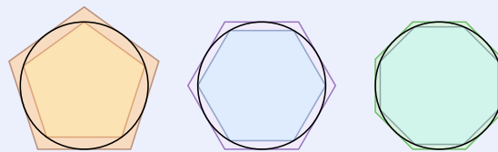
Abbildung 2.4: Schrittweise Annäherung an einen Kreis durch ein- beziehungsweise umbeschriebene regelmässige Polygone (links: 5-Ecke, mittels: 6-Ecke, rechts: 8-Ecke).
